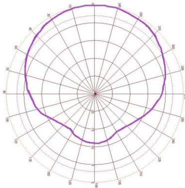
YZ-plane – Vertical Pol
